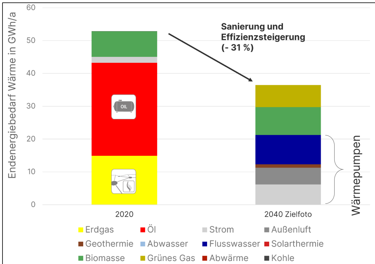
Abbildung 27: Energieträger zur Wärmeversorgung im Basis- und Zieljahr
