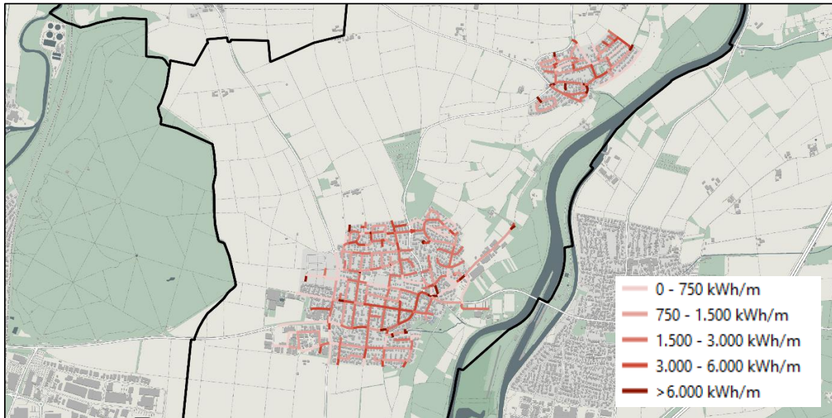
Abbildung 6: Wärmelinien-dichte
