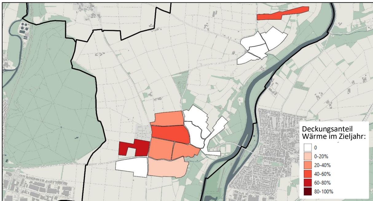
Abbildung 14: Potenzialkarte „Geothermie – Sonden dezentral“ auf Clusterebene
