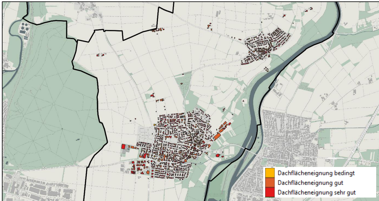
Abbildung 22: Potenzialkarte „Photovoltaik – dezentral“ auf Gebäudeebene (Einstufung nach Energieatlas BW)
