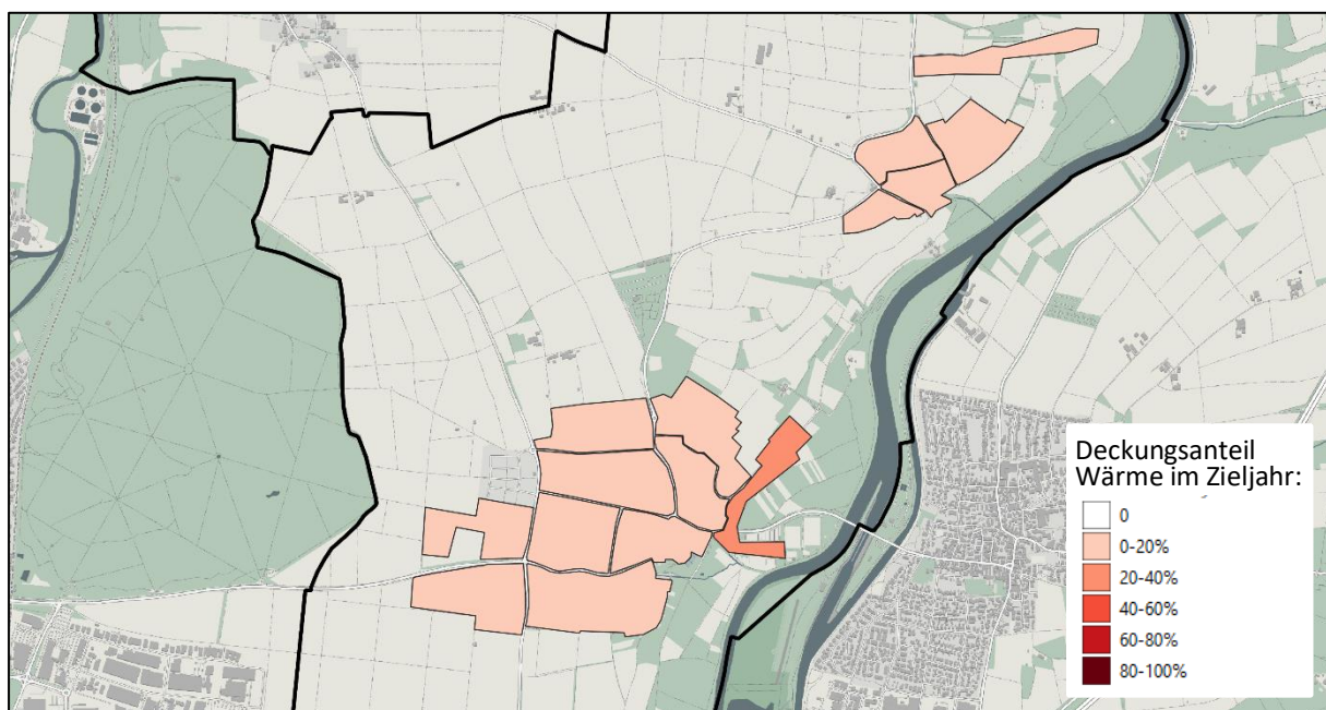
Abbildung 16: Potenzialkarte „Solarthermie - dezentral“ auf Clusterebene
