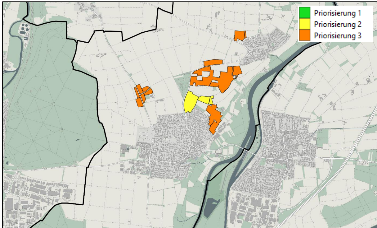
Abbildung 17: Eignungsflächen für das Potenzial „Solarthermie - zentral“
