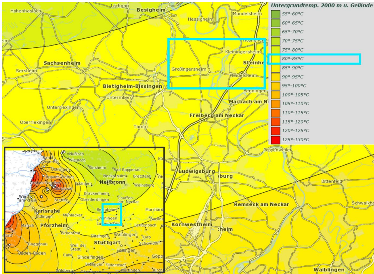
Abbildung 20: Potenzialkarte „Tiefengeothermie“ in 2.000 m
