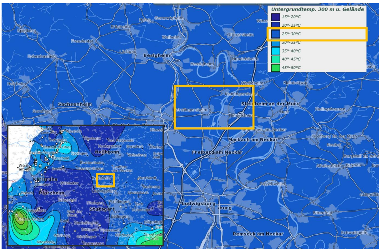
Abbildung 19: Potenzialkarte „Tiefengeothermie“ in 300 m
