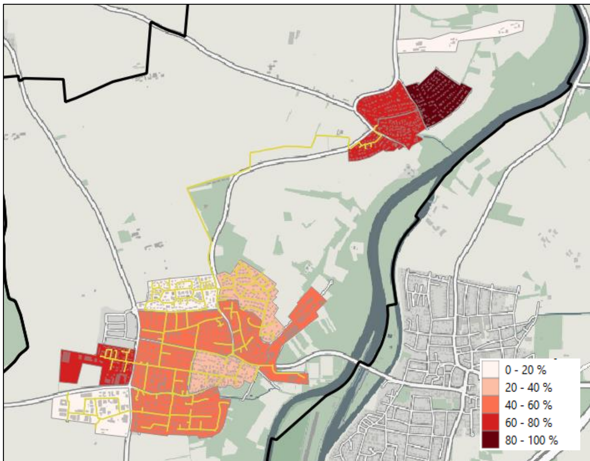
Abbildung 36 Darstellung der Anteile an Öl-Heizungsanlagen je Cluster und Lage des Gasnetzes (gelb) in Ingersheim.
