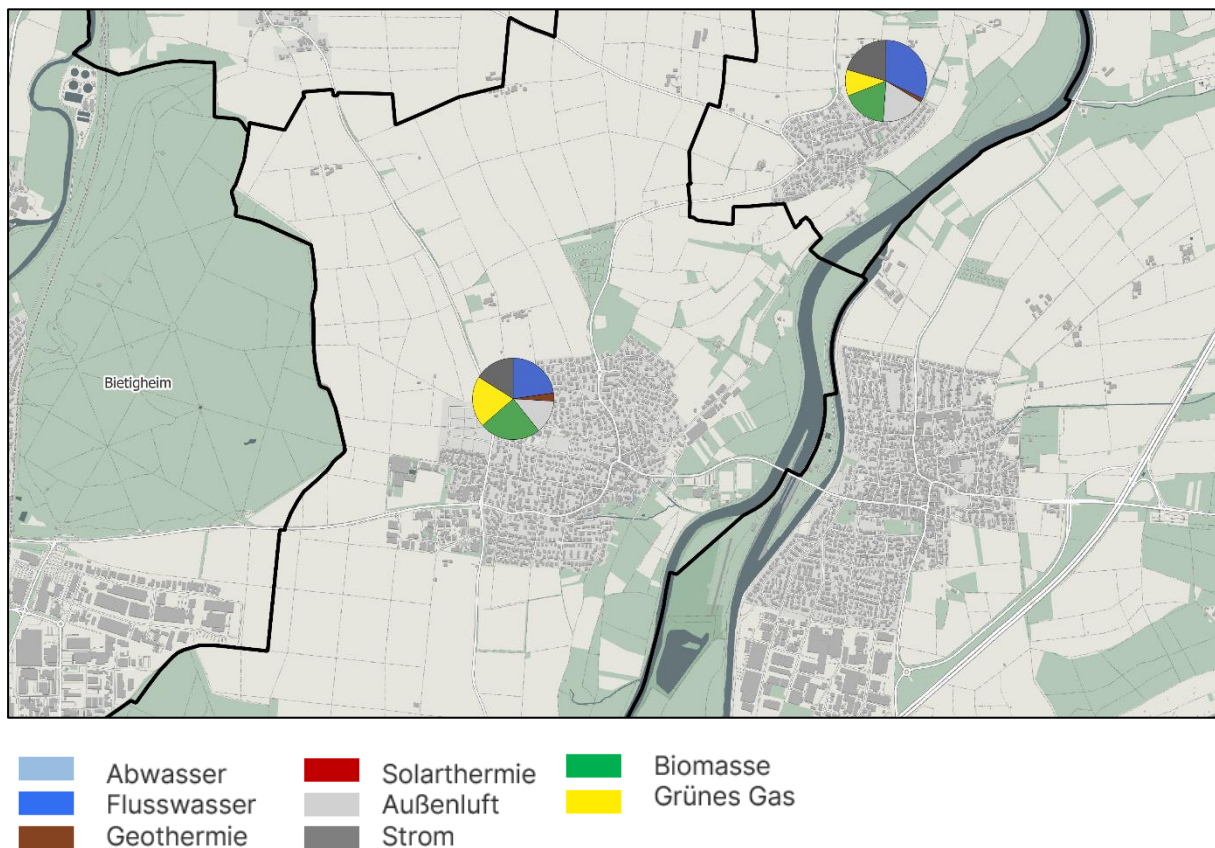
Abbildung 28: Zielfoto 2035 Energieversorgung der Stadtteile
