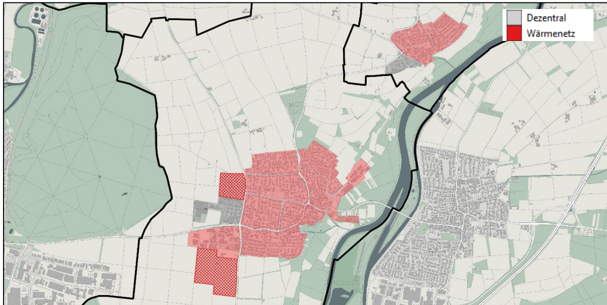
Abbildung 31: Clusterkarte mit Wärmenetzgebieten aus dem Zielfoto
