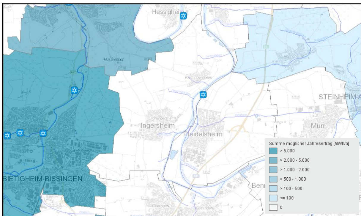
Abbildung 25: Wasserkraftpotenzial aus Energieatlas BW
