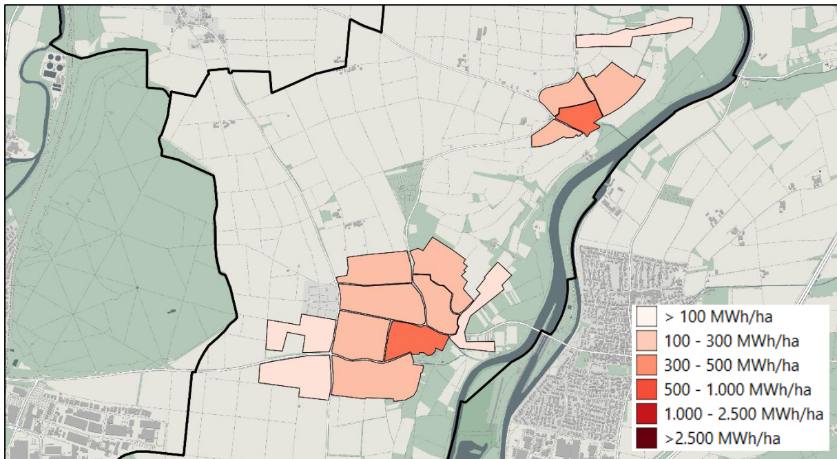
Abbildung 5: Wärmedichte je Cluster
